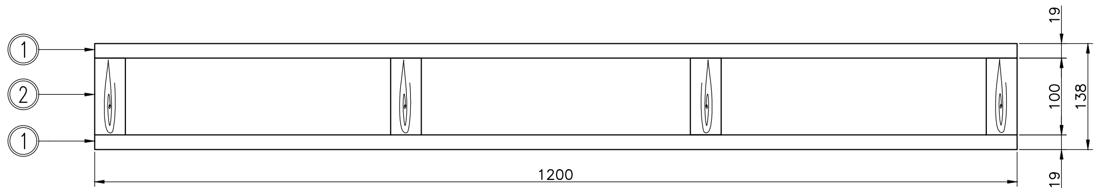
PERSPECTIVA SUPERIOR ESC. 1:5
