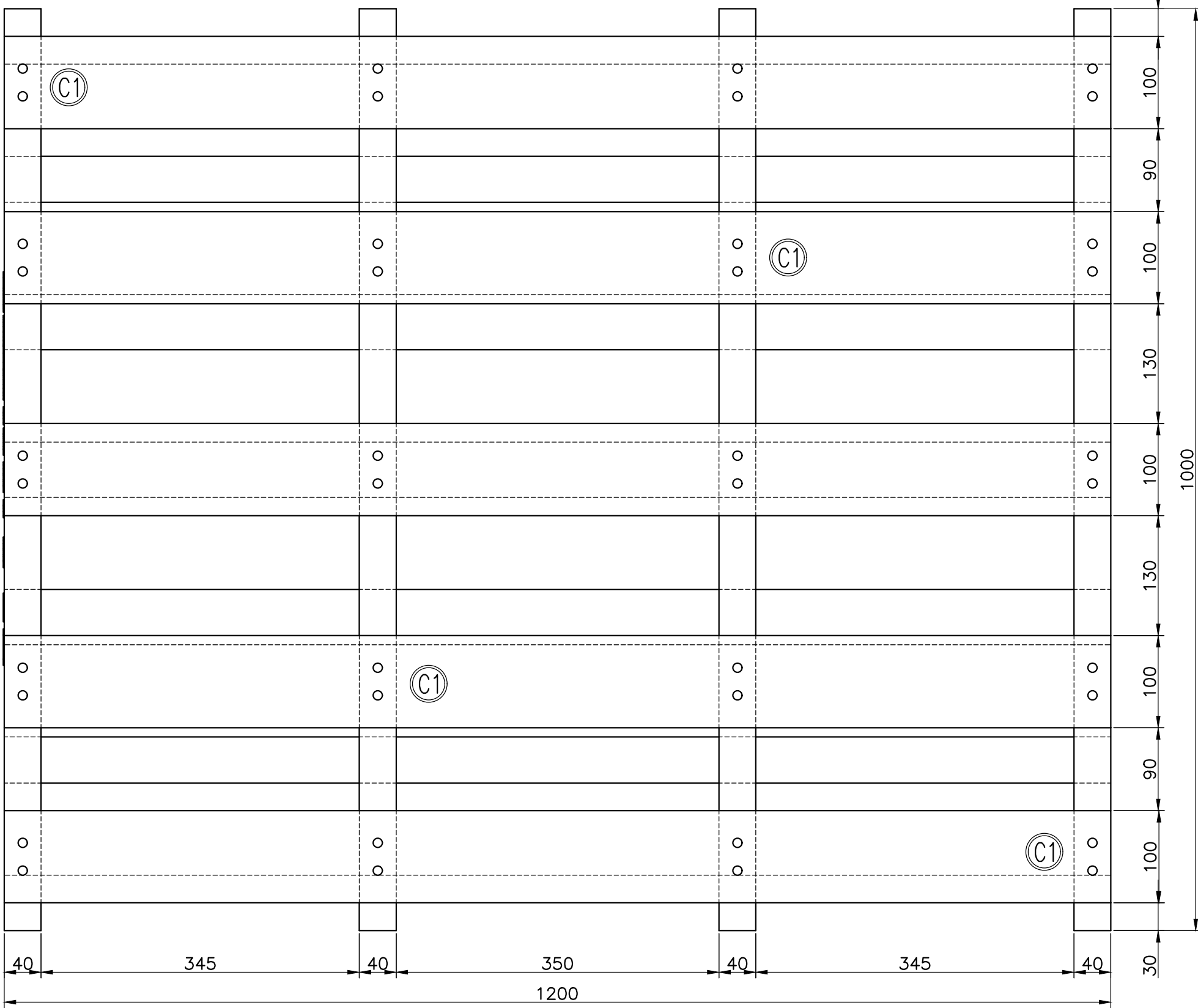
APILADO DE PALLETS ESC. 1:5
