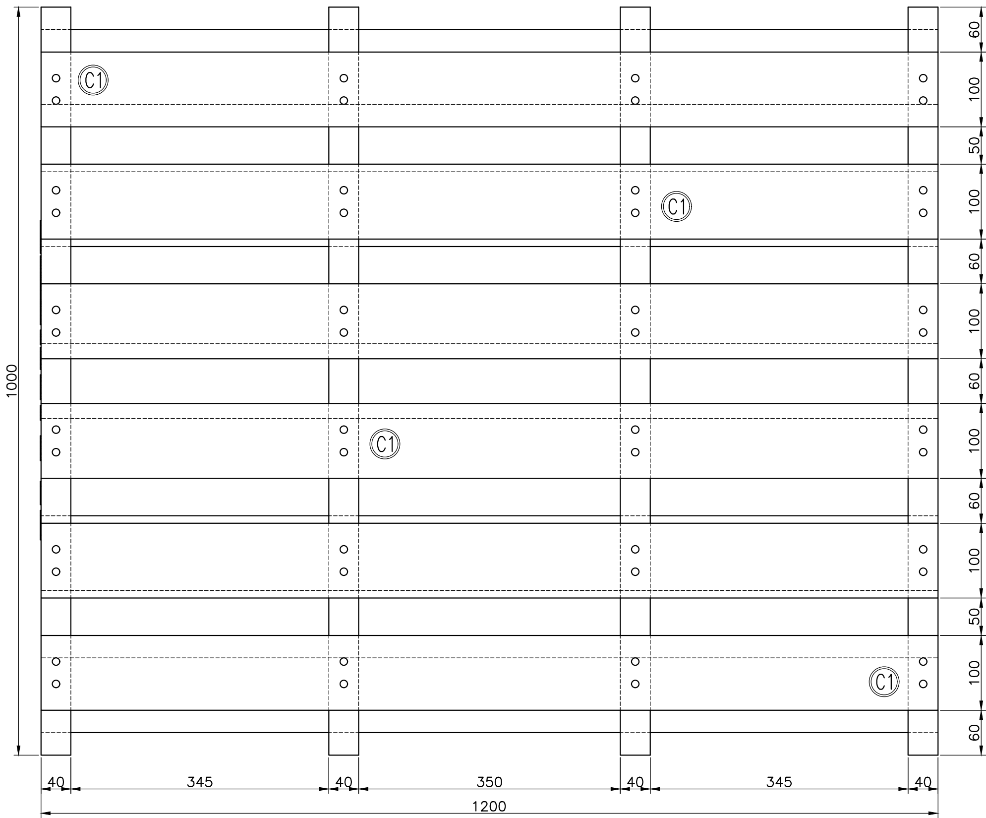
VISTA SUPERIOR ESC. 1:5
